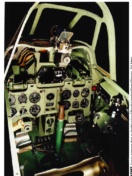
A6M3 (www.aeronautics.ru/archivewww/ibooks/cockpit/small/page_04.htm)
